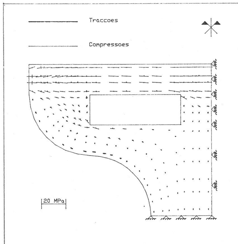
Figura 16 Tensões principais no betão (fase I)
