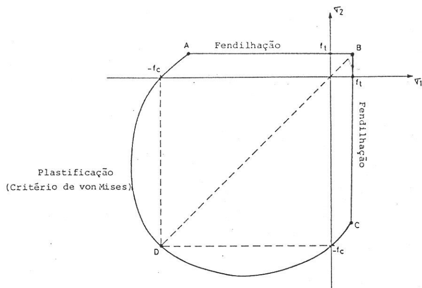
Figura 1 Comportamento bidimensional do betão considerado no modelo matemático
