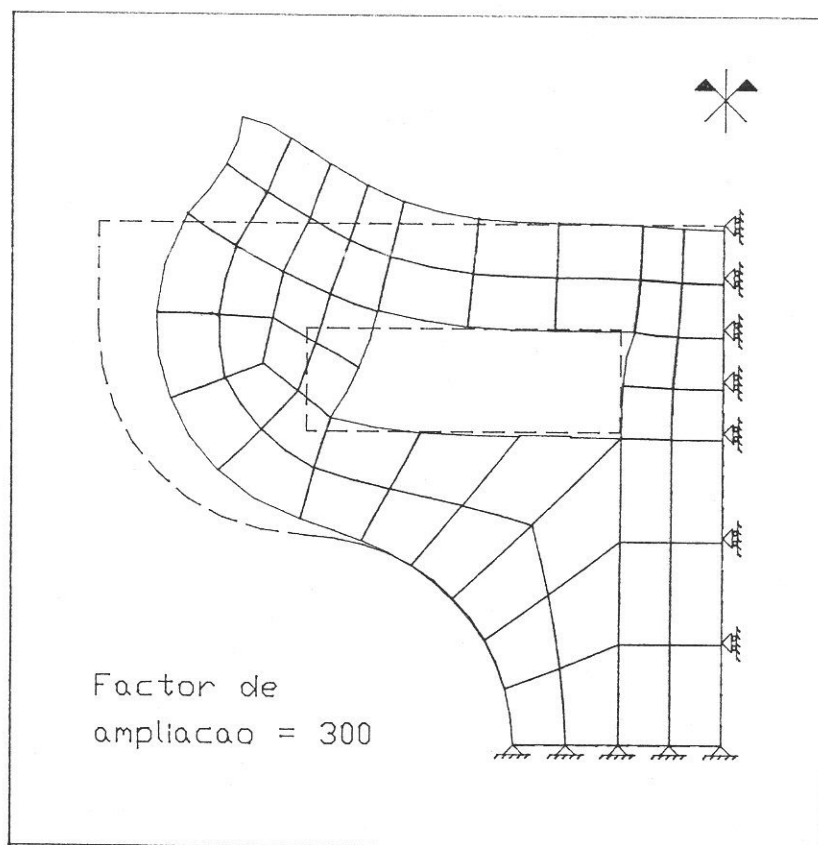
Figura 13 Deslocamentos (fase I)
