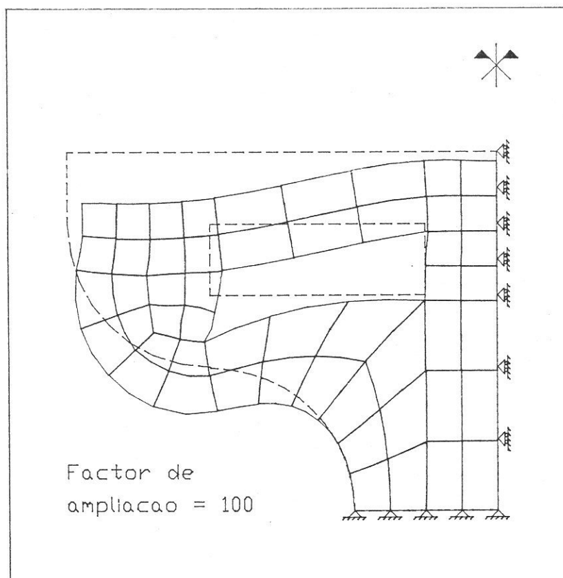
Figura 14 Deslocamentos (fase II)
