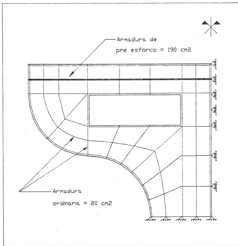
Figura 12 Traçado das armaduras ordinárias e de pré-esforço
