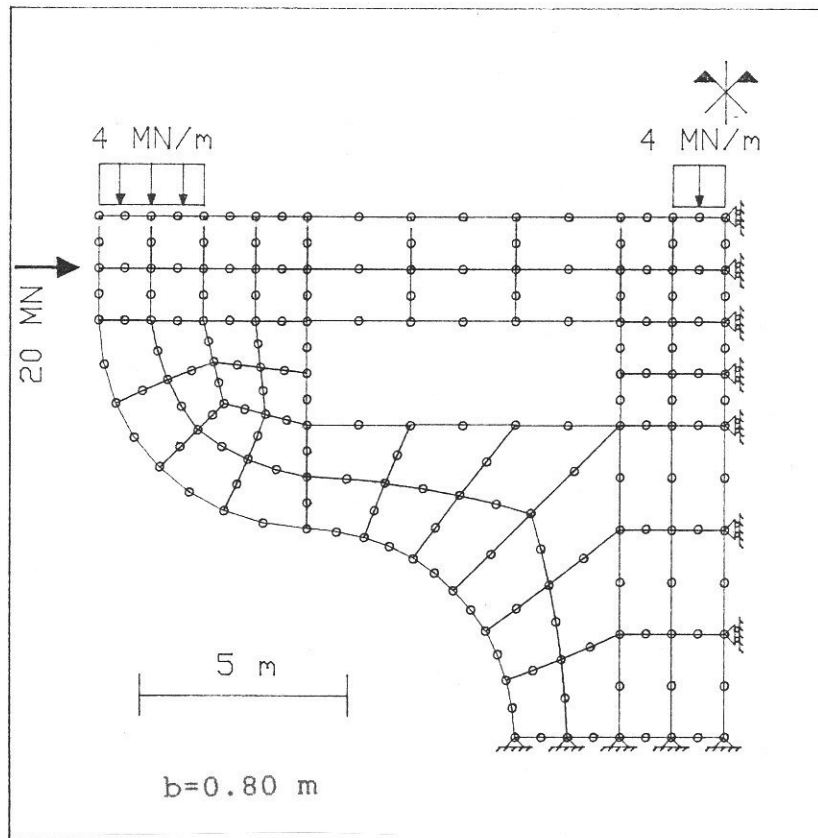
Figura 11 Consola com abertura: malha de elementos finitos e solicitações
