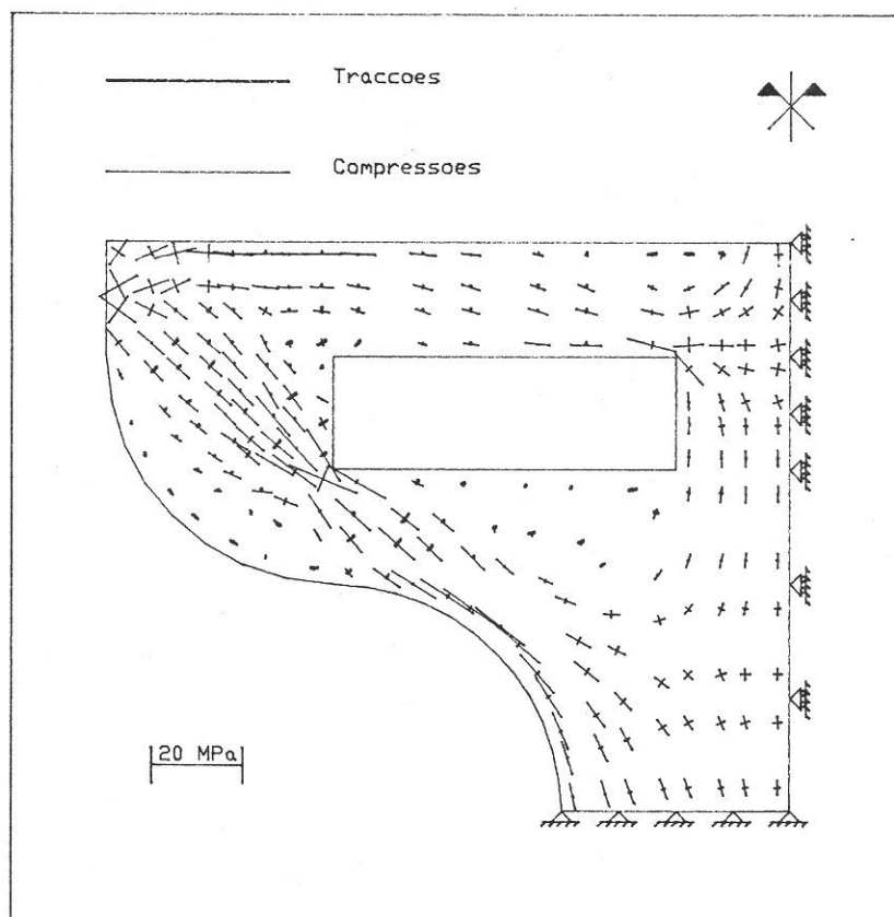
Figura 17 Tensões principais no betão (fase II)
