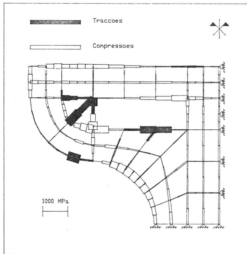
Figura 19 Tensões na armadura (fase II)
