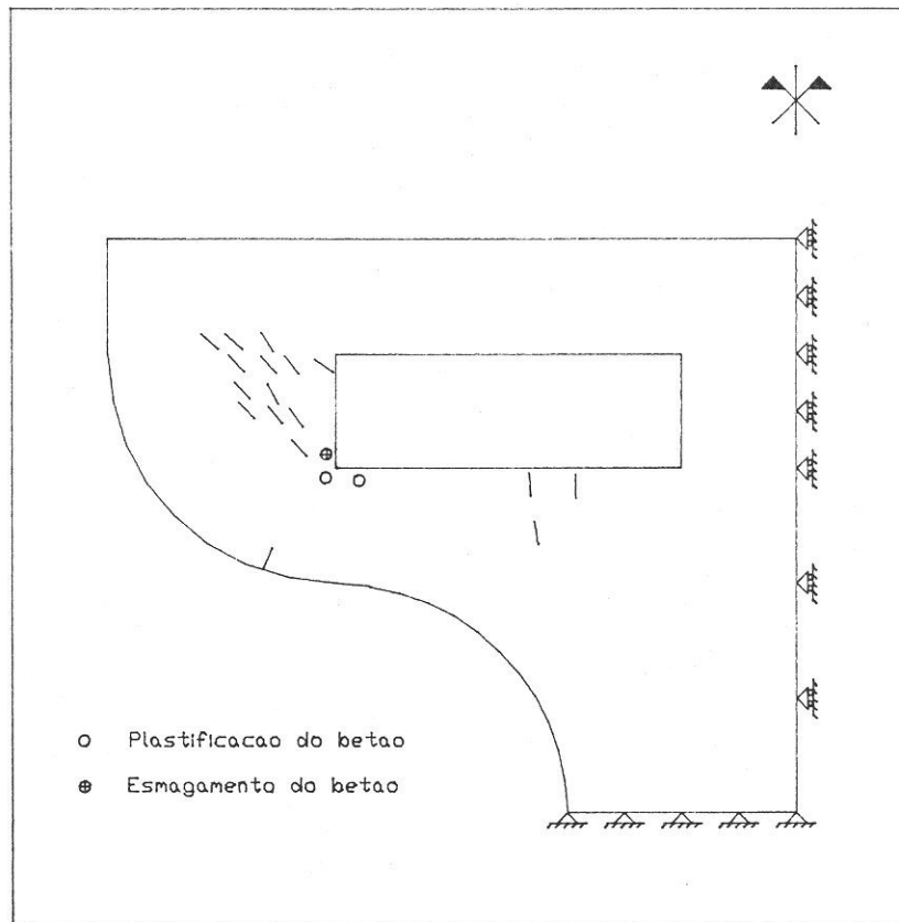
Figura 15 Localização das fendas e das zonas plastificadas (fase II)
