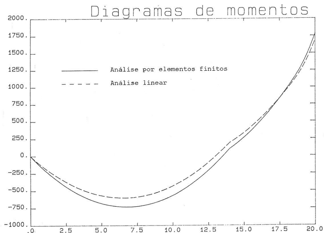
Figura 8 Diagramas de momentos obtidos na análise linear e e na análise não linear
