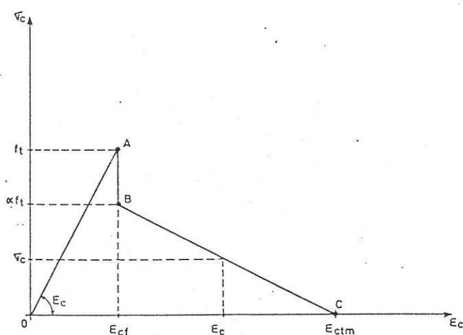
Figura 2 Diagrama tensões-deformações do betão fendilhado
