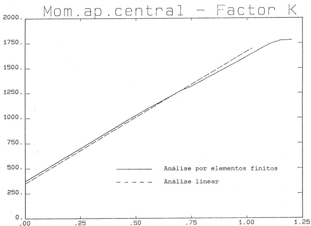
Figura 9 Diagramas momentos-factor factor de carga K obtidos na análise linear e na análise não linear
