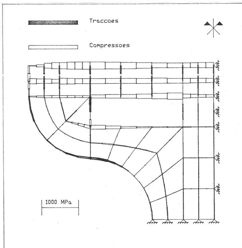
Figura 18 Tensões na armadura (fase I)
