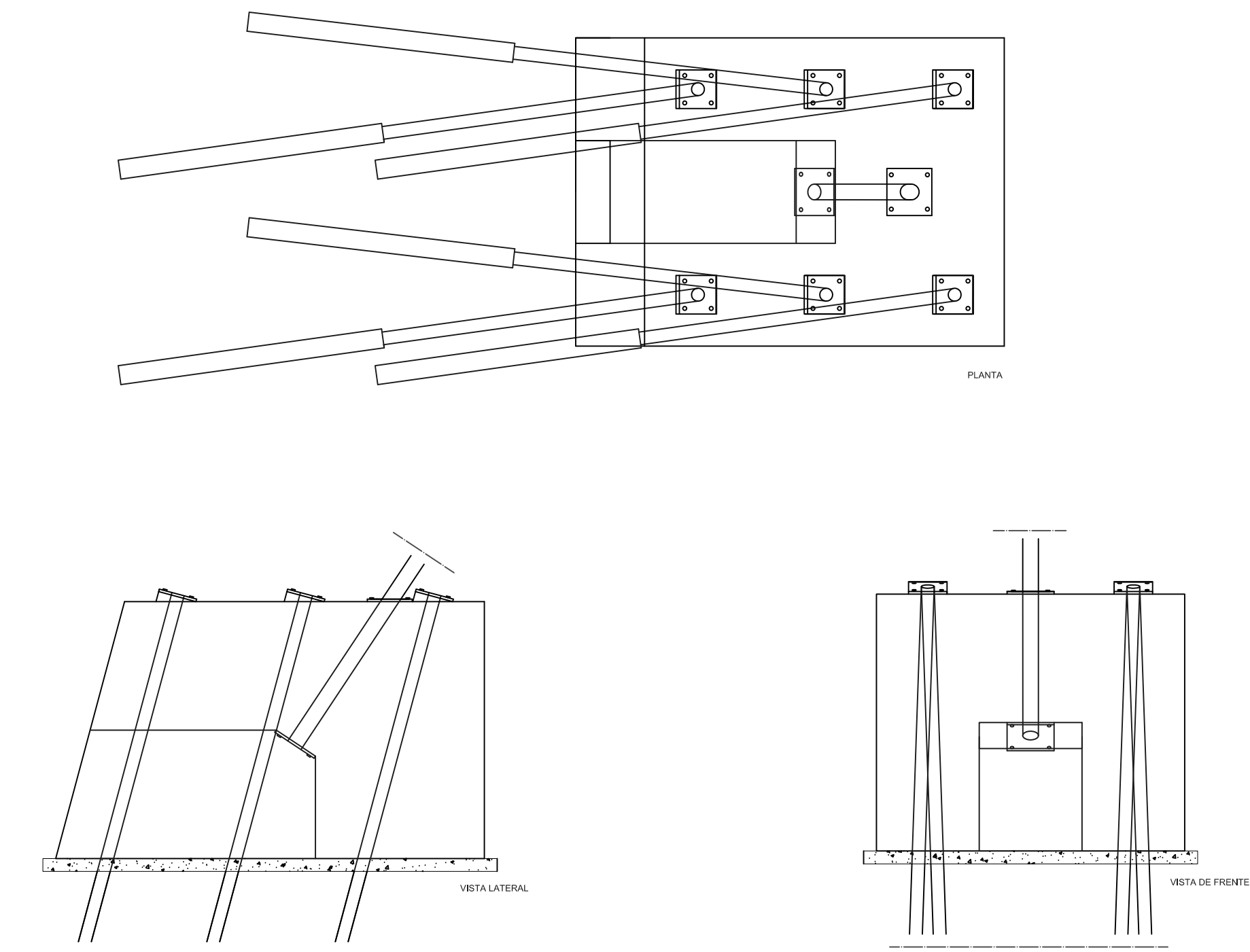
Maciço de fundação das ancoragens - cabos exteriores
