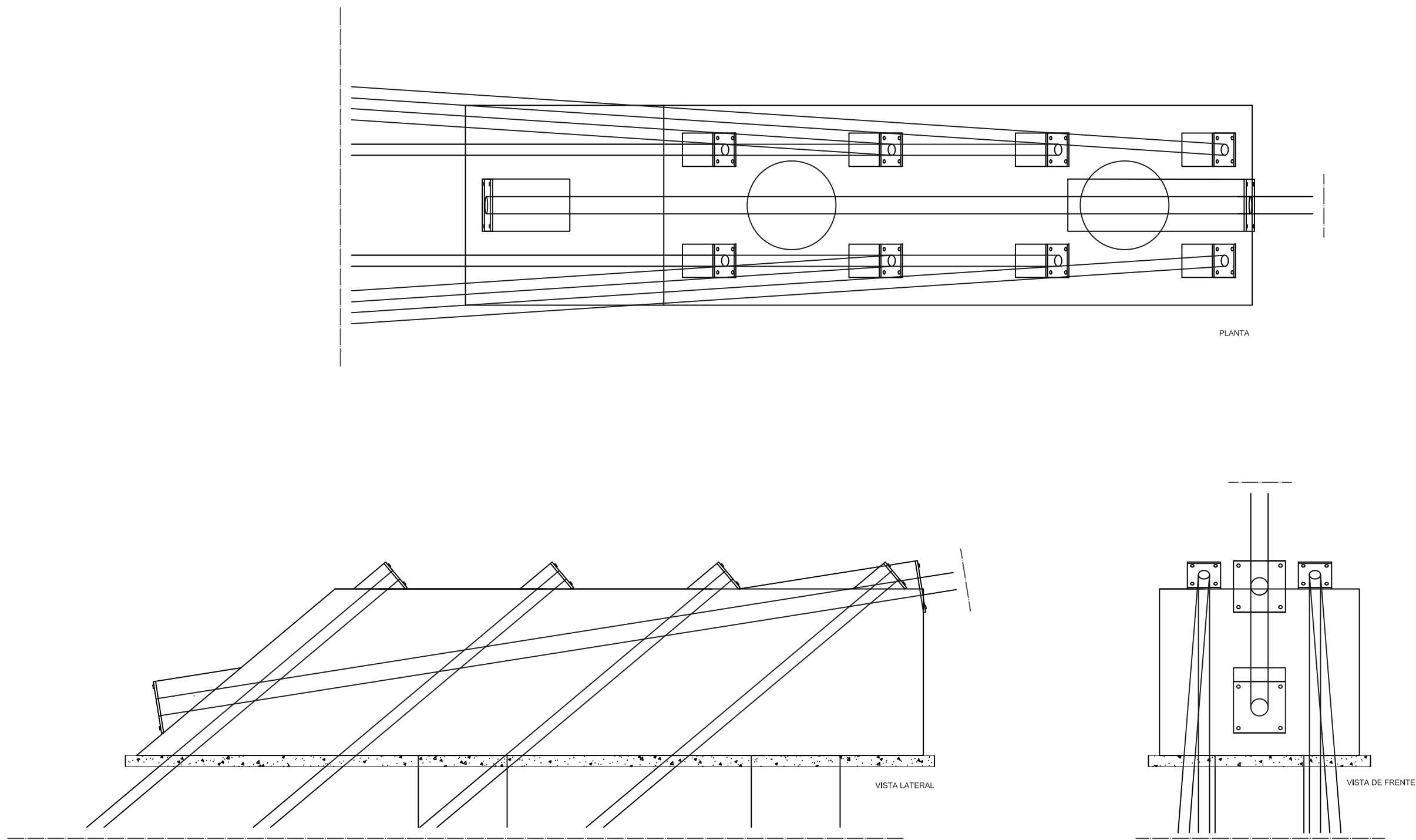
Maciço de fundação das ancoragens - cabos inferiores
